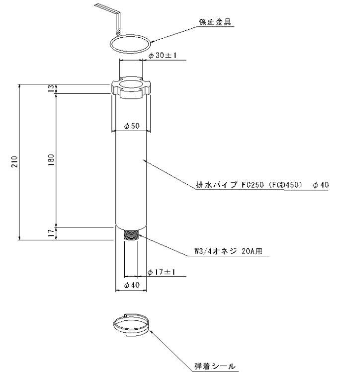
排水パイプ詳細図(T-210)
